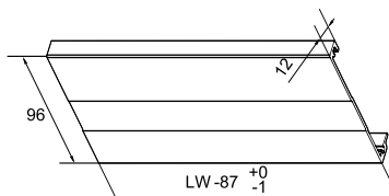
Крепление фасада
