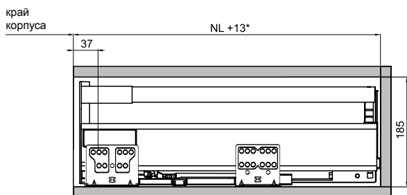
Ящик внутренний
